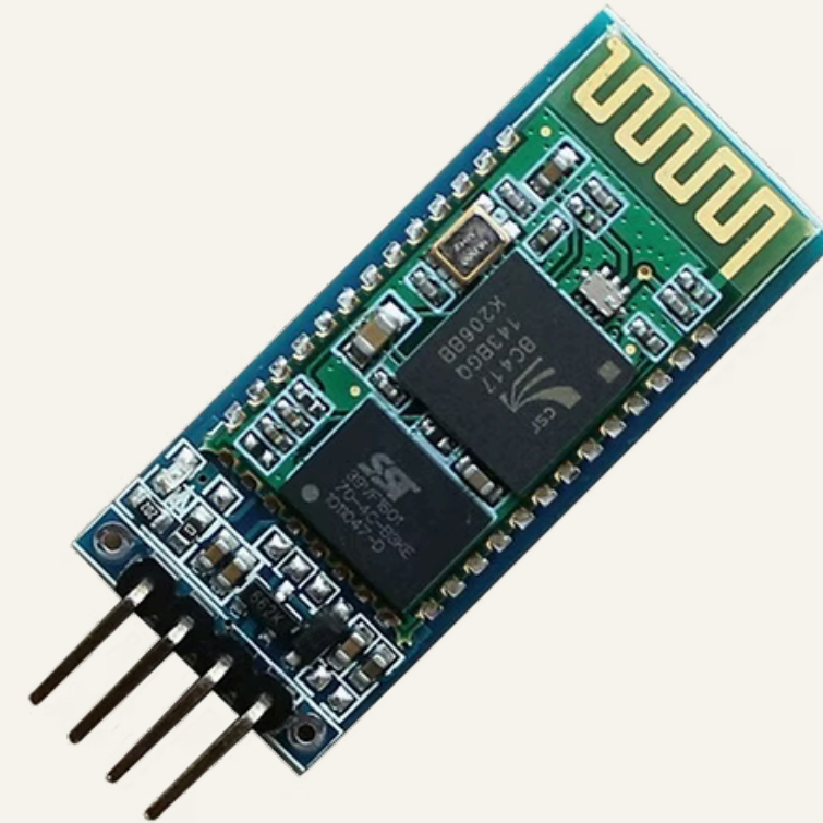
6 HC-06 Bluetooth Module
