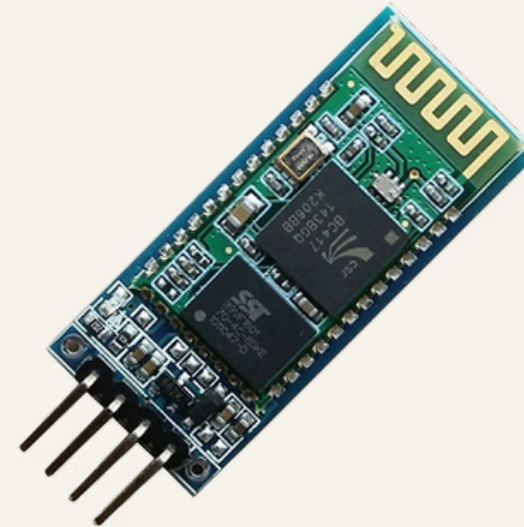
HC-06 Bluetooth Module
